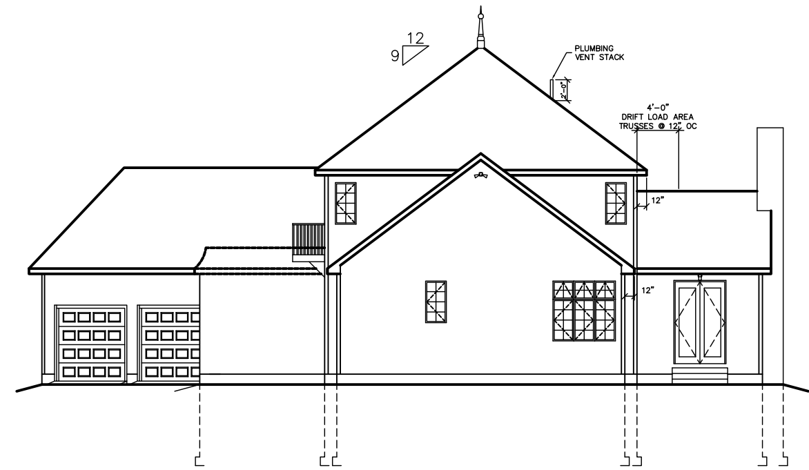
RIGHT ELEVATION
